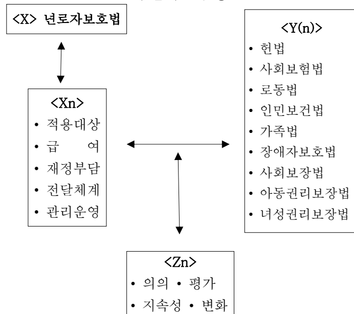
〈그림 1〉 분석모형
